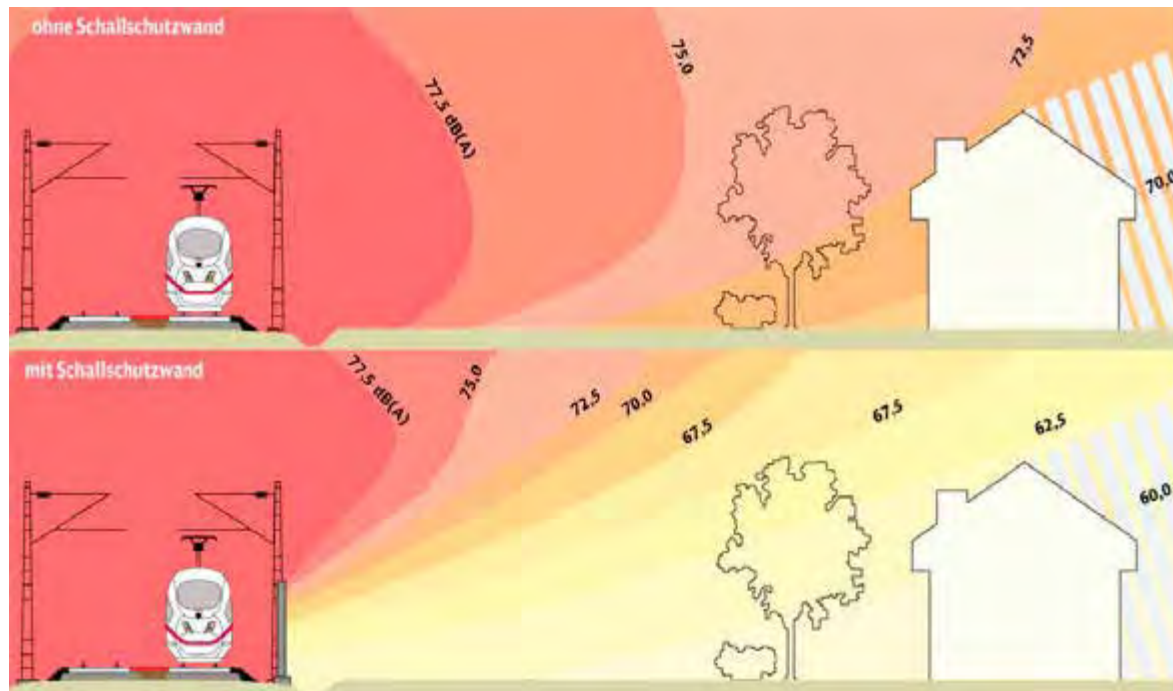
Grafik 2: Darstellung der Schallausbreitung an Schienen
